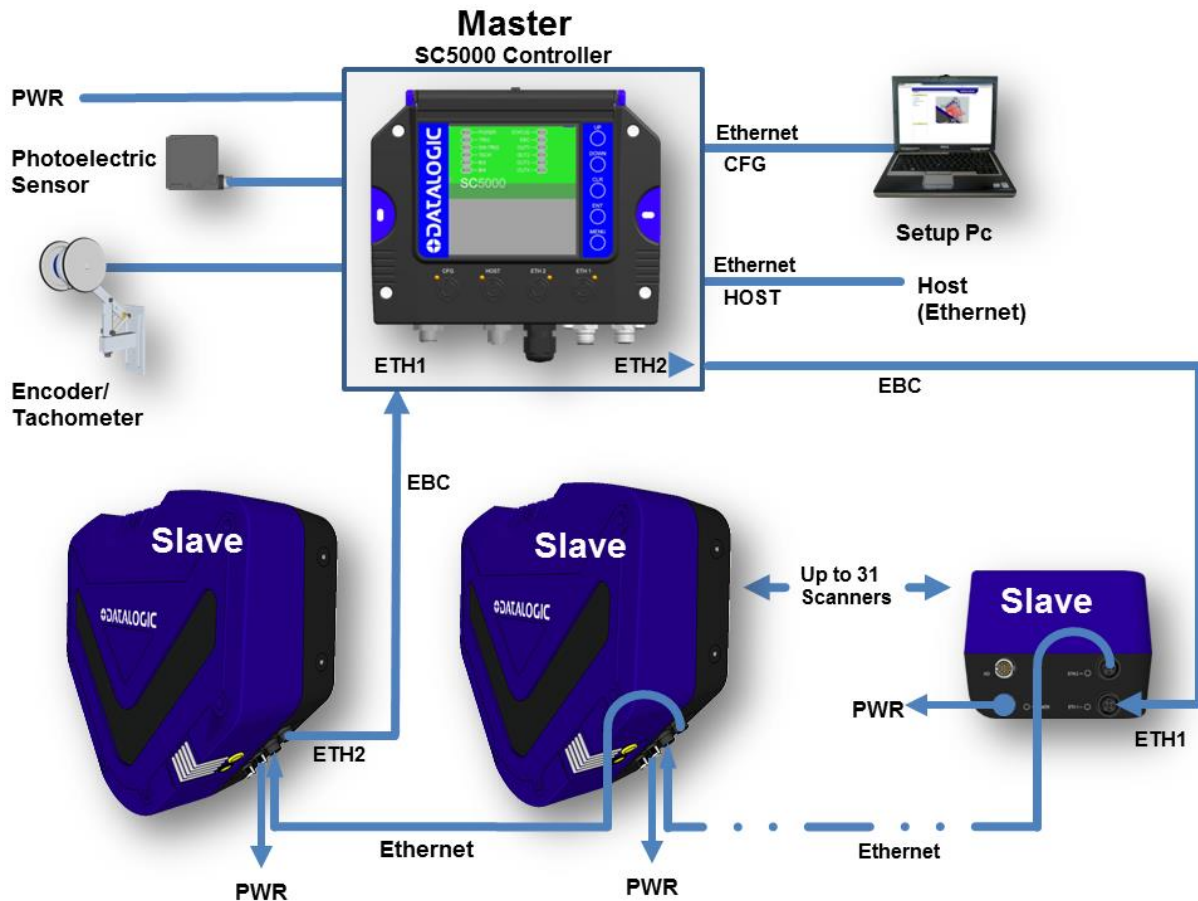
Abb. 19: DX8210-Array (Lesetunnel) mit SC5000 Controller
