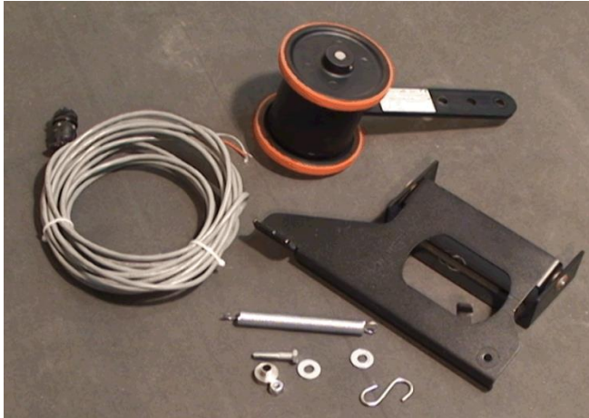
Abb. 7: Drehgeber, Befestigungswinkel und Kabel
