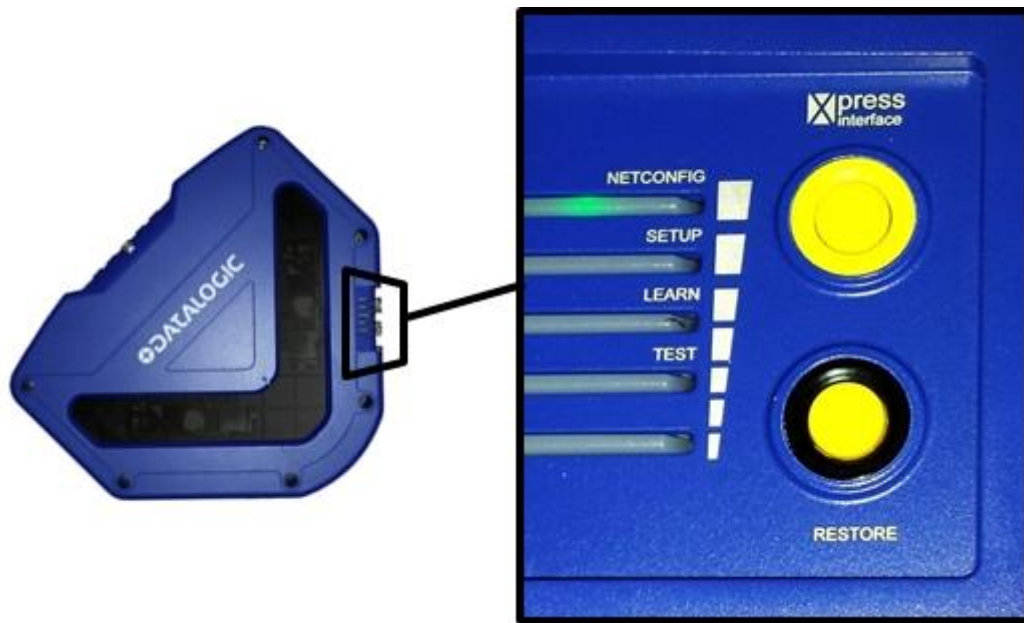
Abb. 37: Tasten des Bediengeräts
