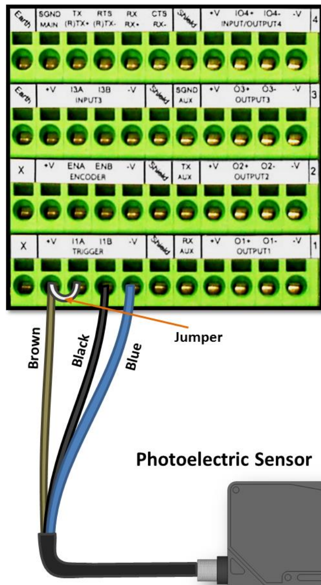
Abb. 24: Kabelanschlüsse des optoelektronischen Sensors (NPN-Ausgang)
