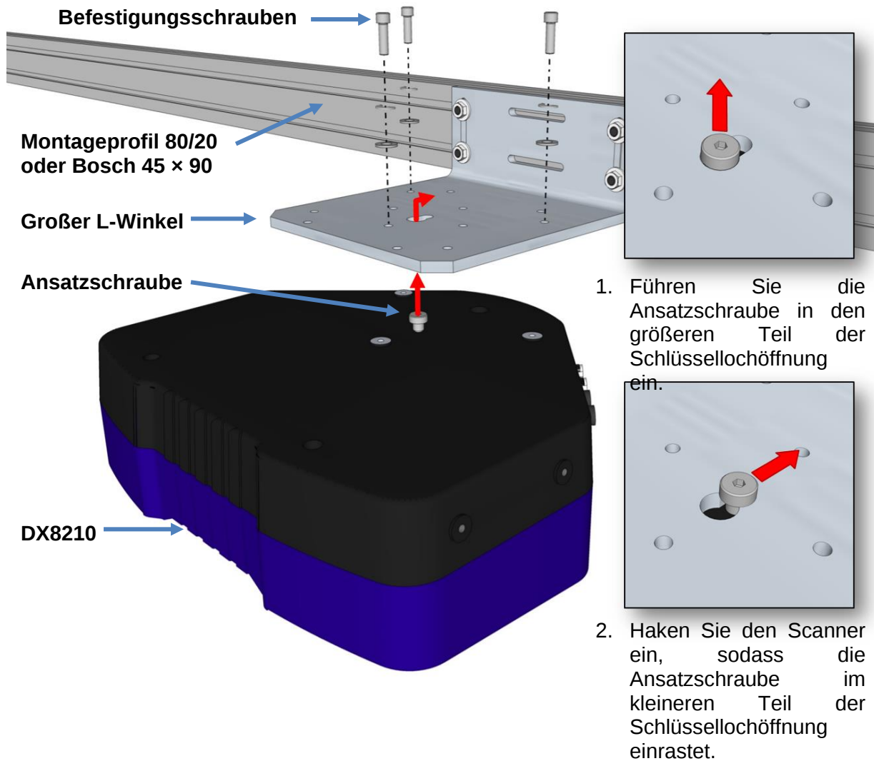
Abb. 15: Einhaken in der Schlüssellochöffnung des großen L-Winkels (Montageprofil 80/20 oder Bosch 45 × 90)
