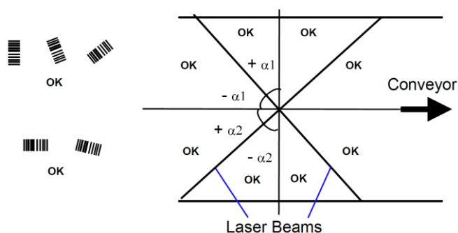
Abb. 73 – Lesebereiche zwischen sich kreuzenden Laserstrahlen mit \alpha_{\max}
