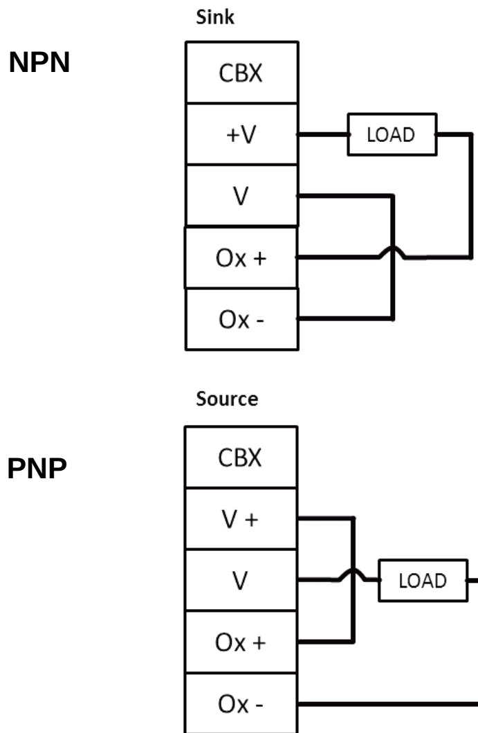
Abb. 32: Ausgänge mit anliegender Spannung
