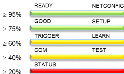
Abb. 39: Leserate (in Prozent) im Testmodus der X-Press Benutzerschnittstelle
