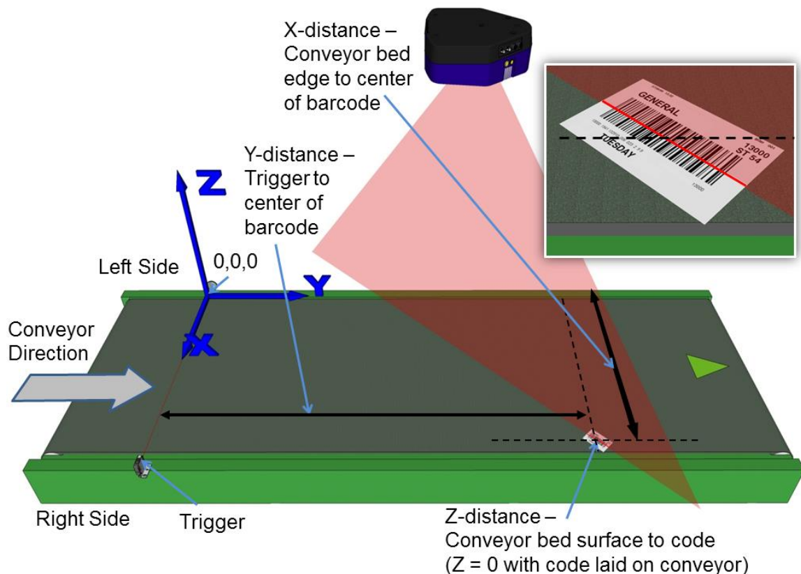
Abb. 49: Platzierung des dritten Barcodes bei oberhalb montiertem Scanner (Laserstrahl 2)
