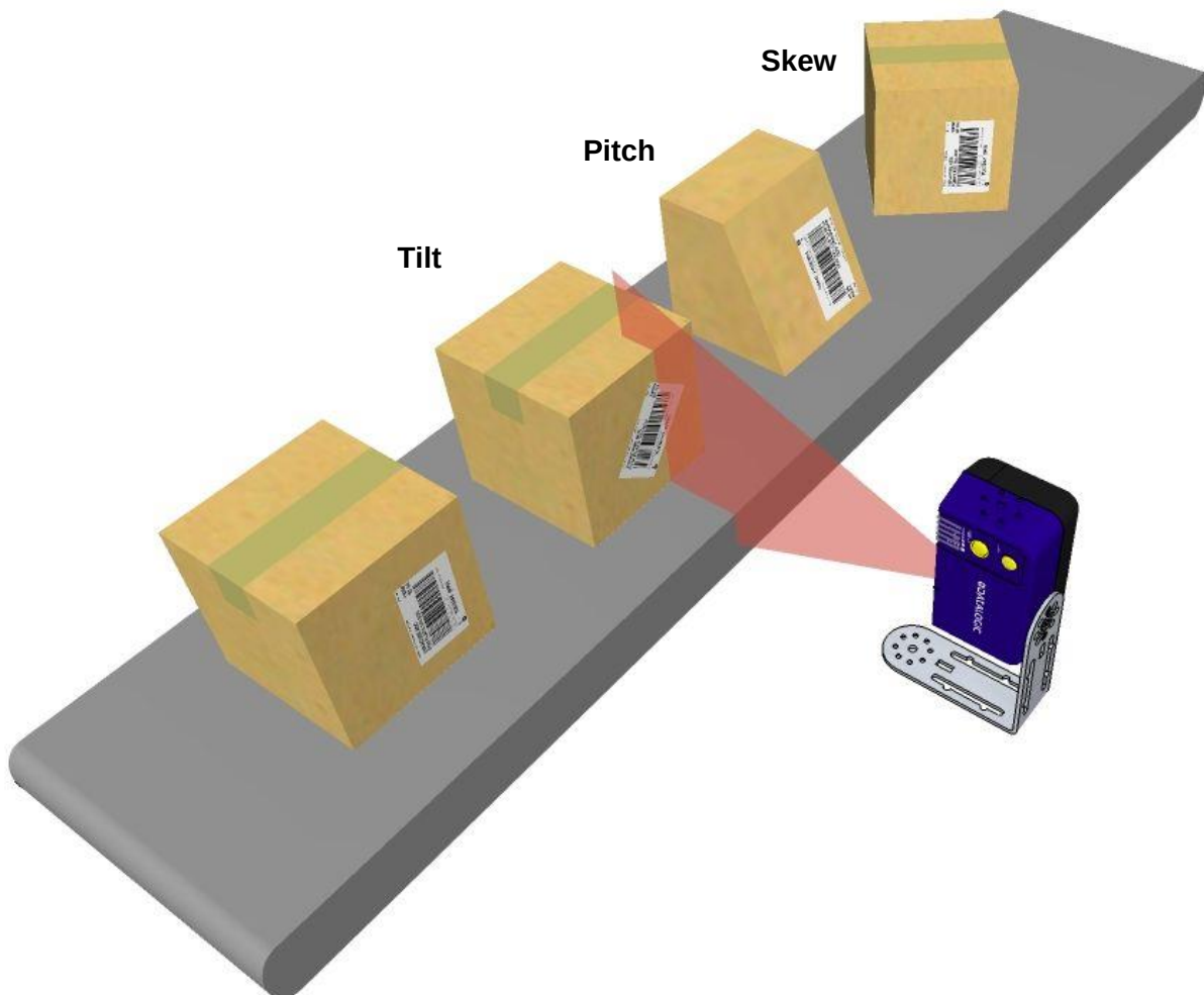
Abb. 18: Kippwinkel (Pitch), Drehwinkel (Skew) und Azimutwinkel (Tilt)
