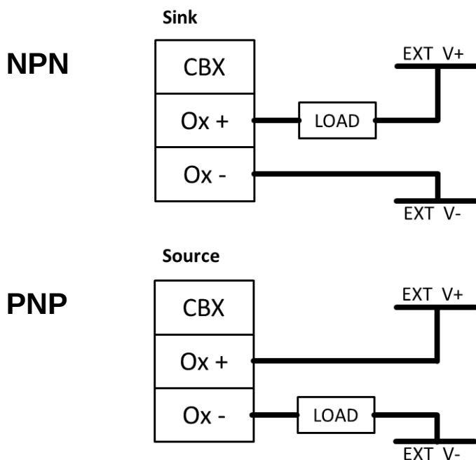
Abb. 33: Ausgänge ohne anliegende Spannung
