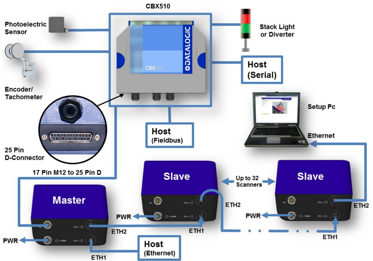
Abb. 20: Master/Slave-Array (Lesetunnel) mit CBX510
