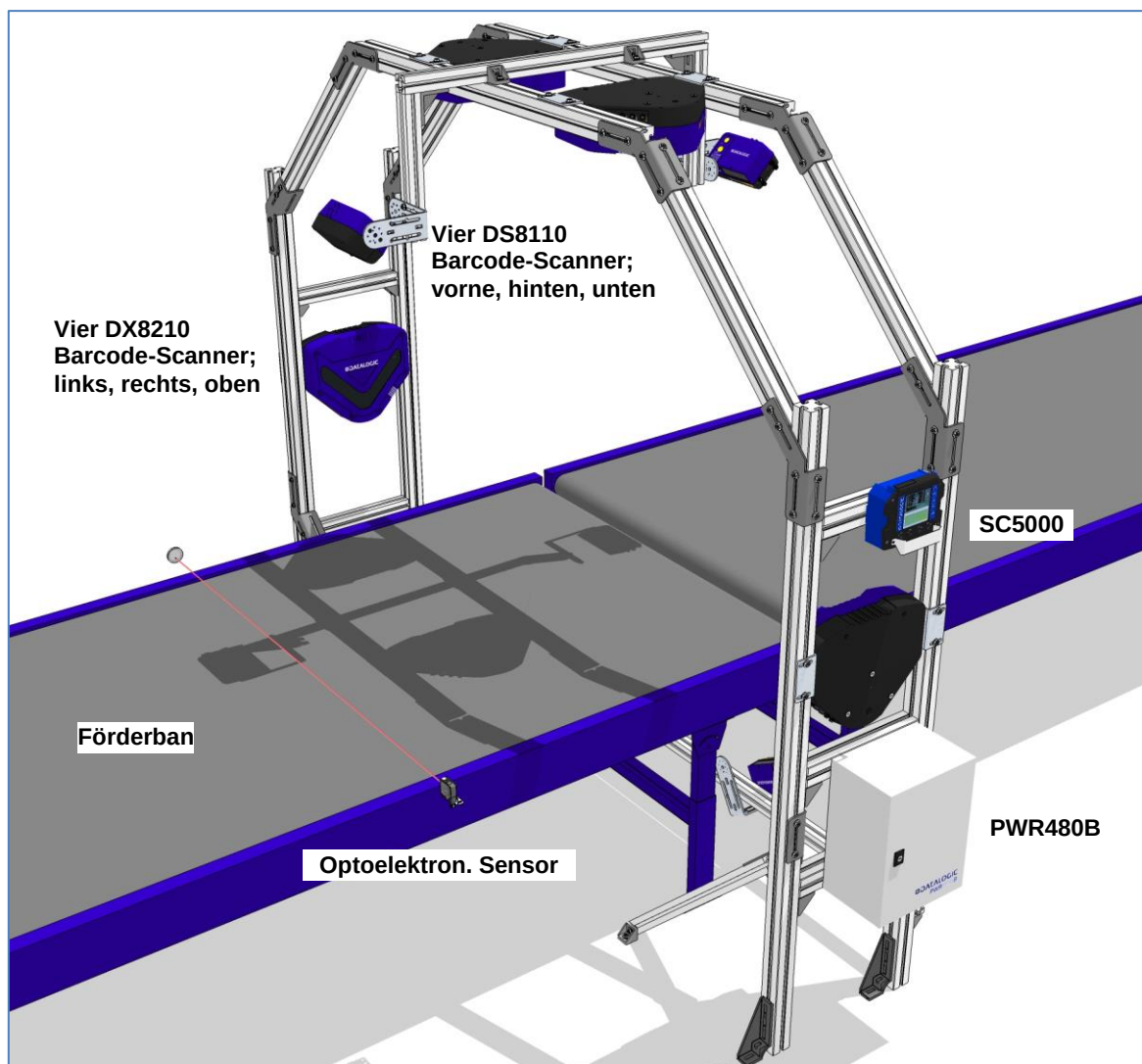
Abb. 55 – Beispiel für eine ATR Lesestation mit großem synchronisierten Netzwerk
